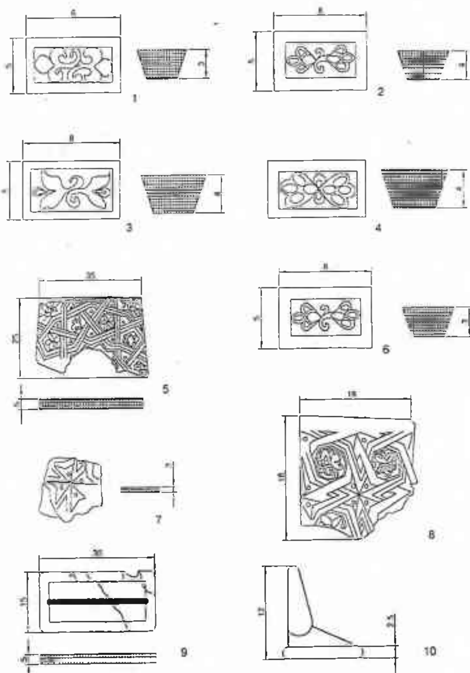
Сурет 3. Қима 5. Шеберханадан шыққан сәулет заттары.
